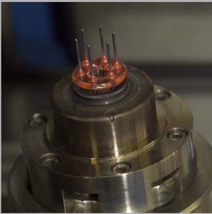
Stromdurchführung
